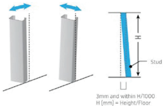
A. Frame vertical unevenness
